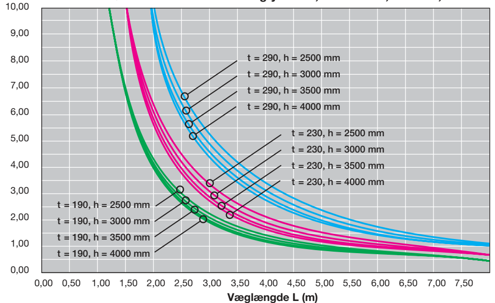
Vandret bæreevne q_{Rd} (kN/m 2 ) Vægtykkelse, t = 190 mm, 230 mm, 290 mm
