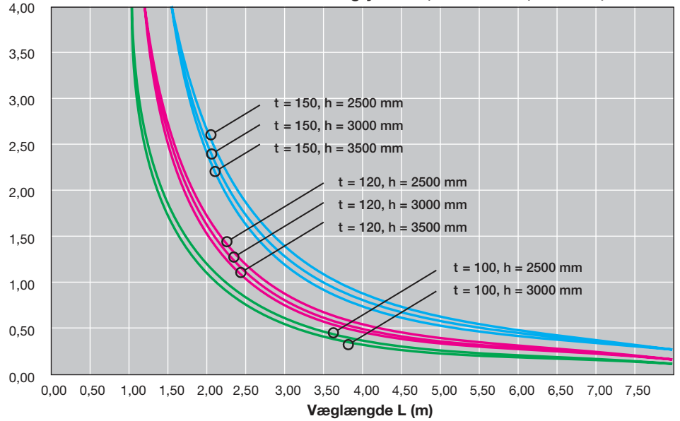
Vandret bæreevne q_{Rd} (kN/m 2 ) Vægtykkelse, t = 100 mm, 120 mm, 150 mm
