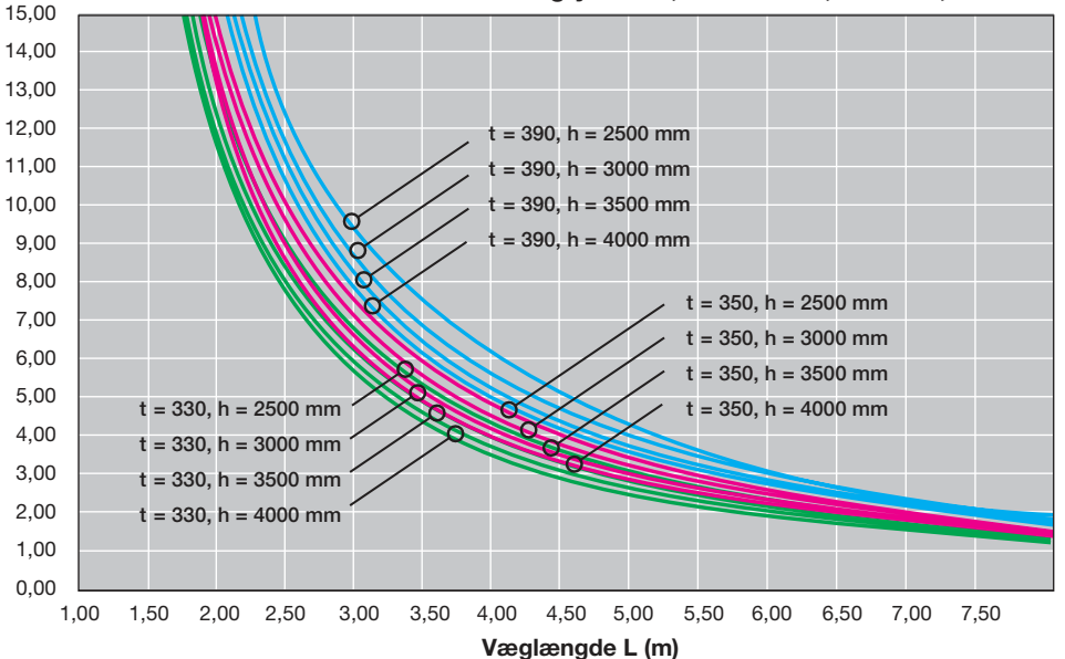
Vandret bæreevne q_{Rd} (kN/m 2 ) Vægtykkelse, t = 330 mm, 350 mm, 390 mm
