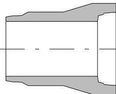
Anboringsmuffe
