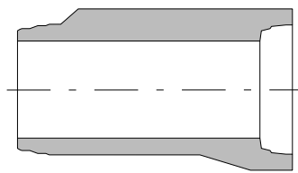
Pasrør
